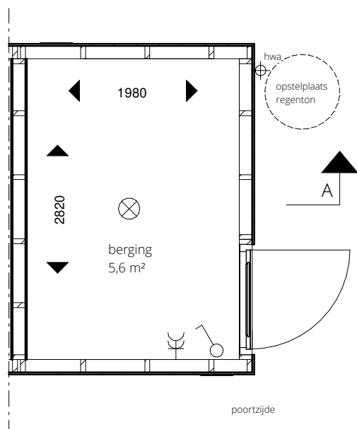
begane grond
