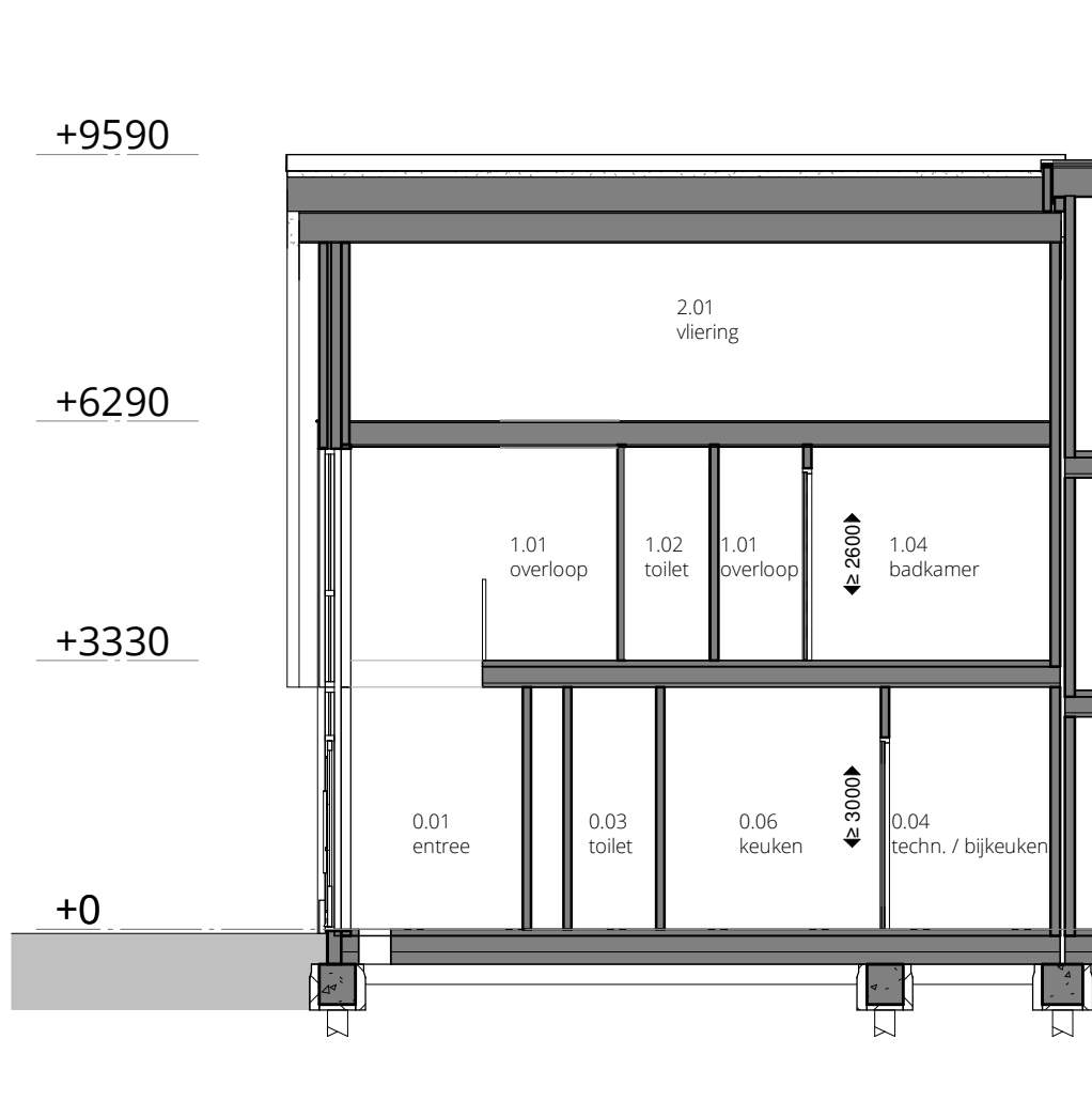
doorsnede A-A
