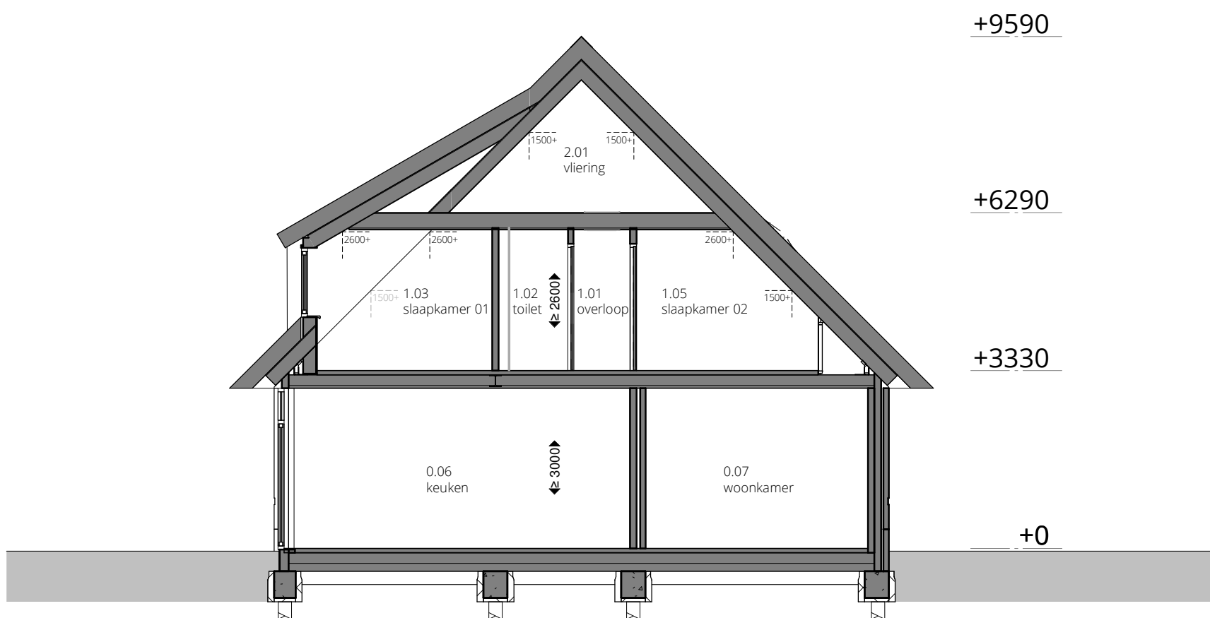
doorsnede B-B
