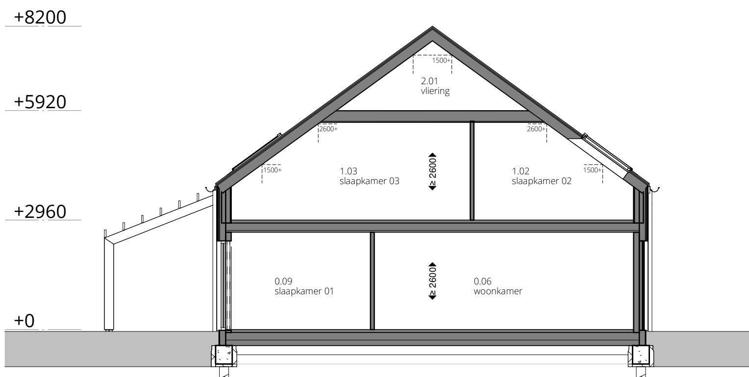
doorsnede C-C
