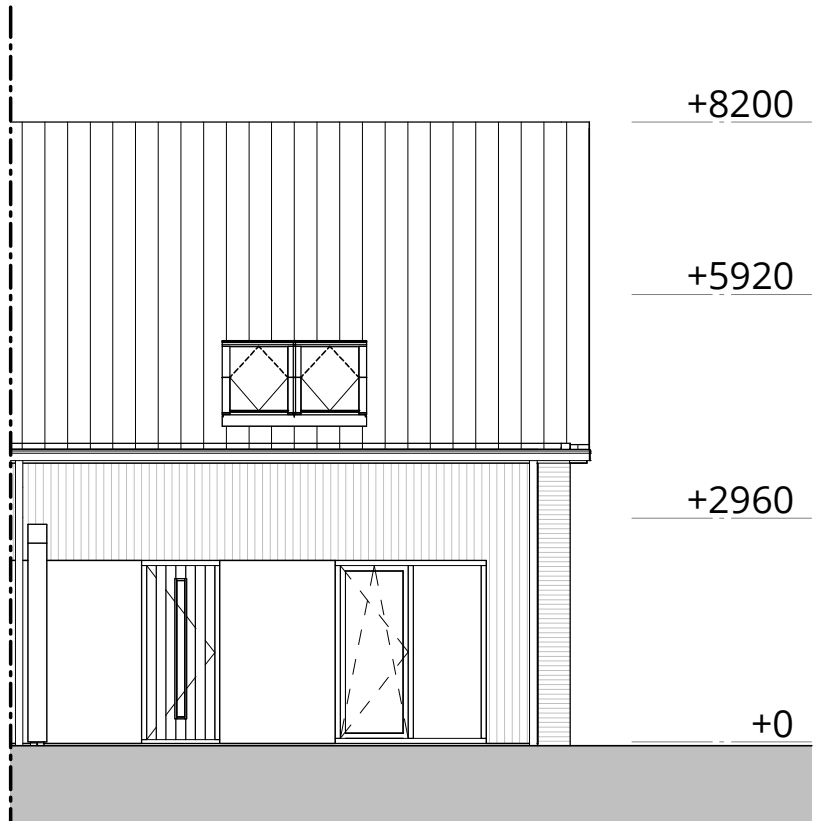
noordoost gevel
