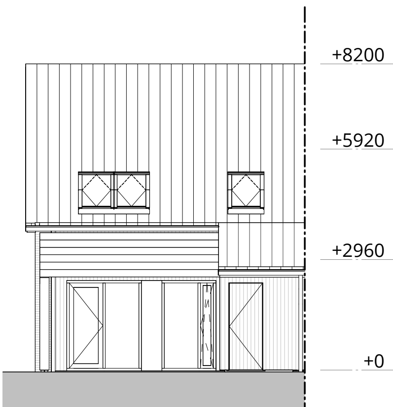
zuidwest gevel
