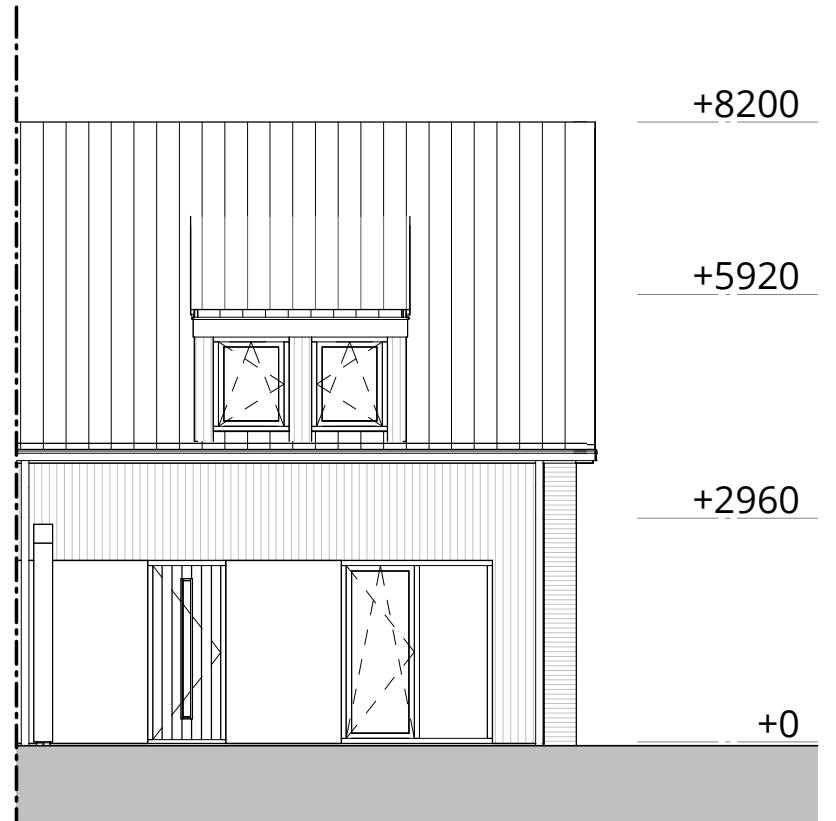
noordoost gevel - optie dakkapel
