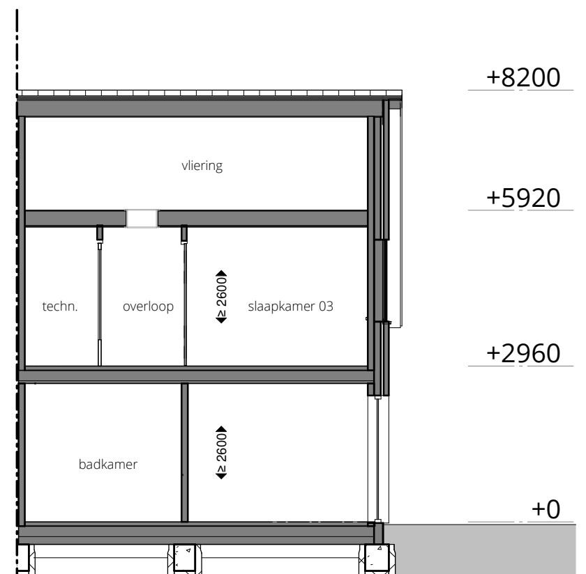
doorsnede A-A
