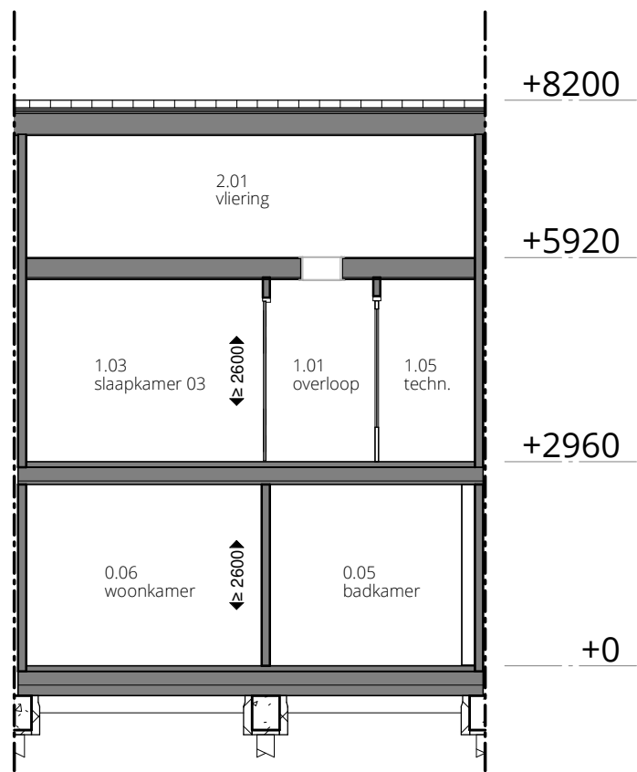
doorsnede A-A
