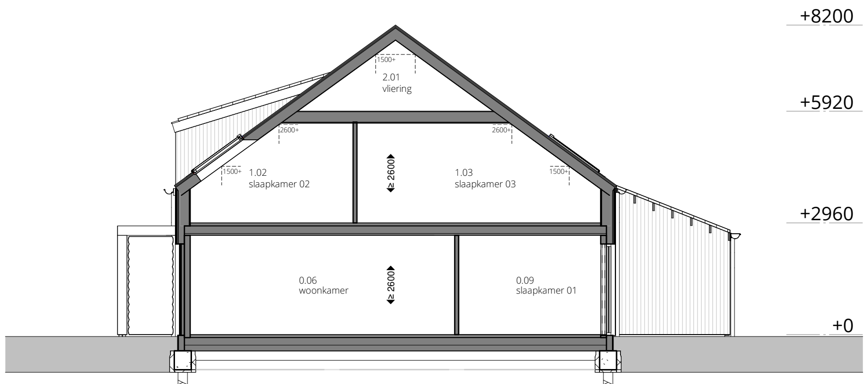
doorsnede B-B
