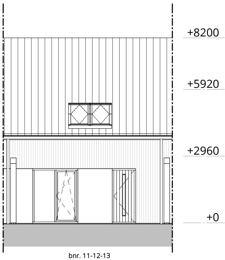
noordoost gevel
