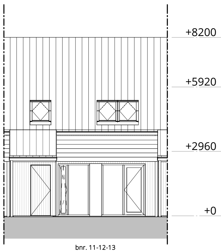
zuidwest gevel
