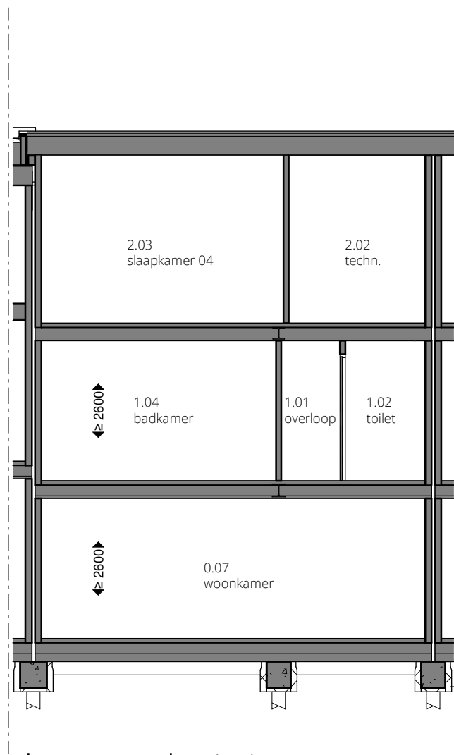
doorsnede A-A
