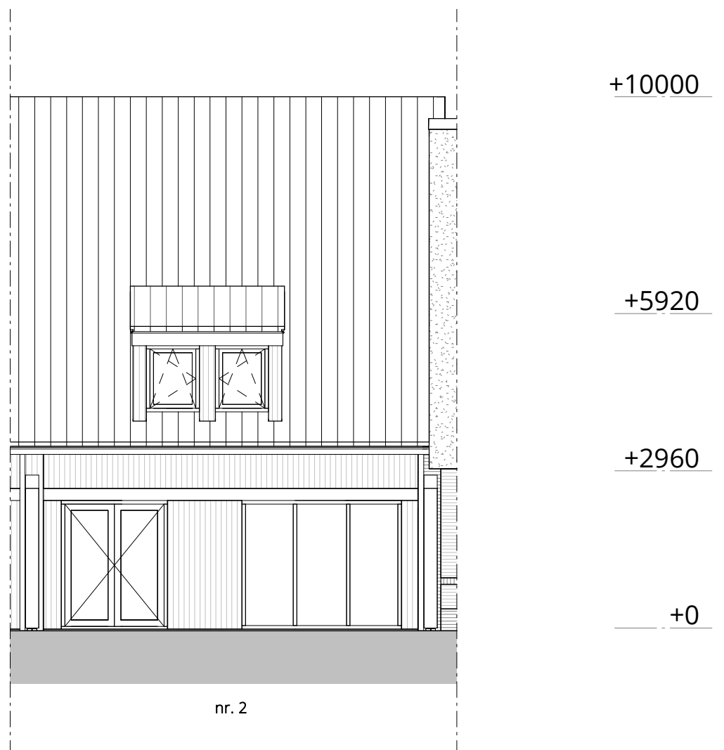
zuidwest gevel - optie dakkapel
