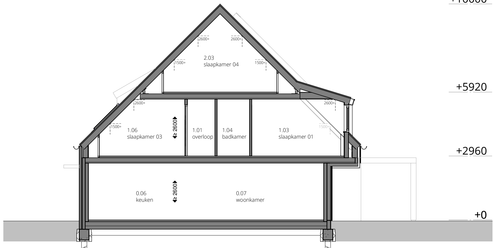
doorsnede C-C - optie dakkapel
