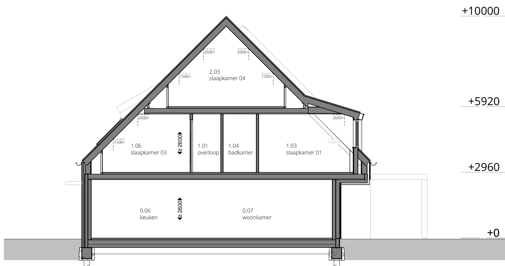
doorsnede C-C - optie dakkapel
