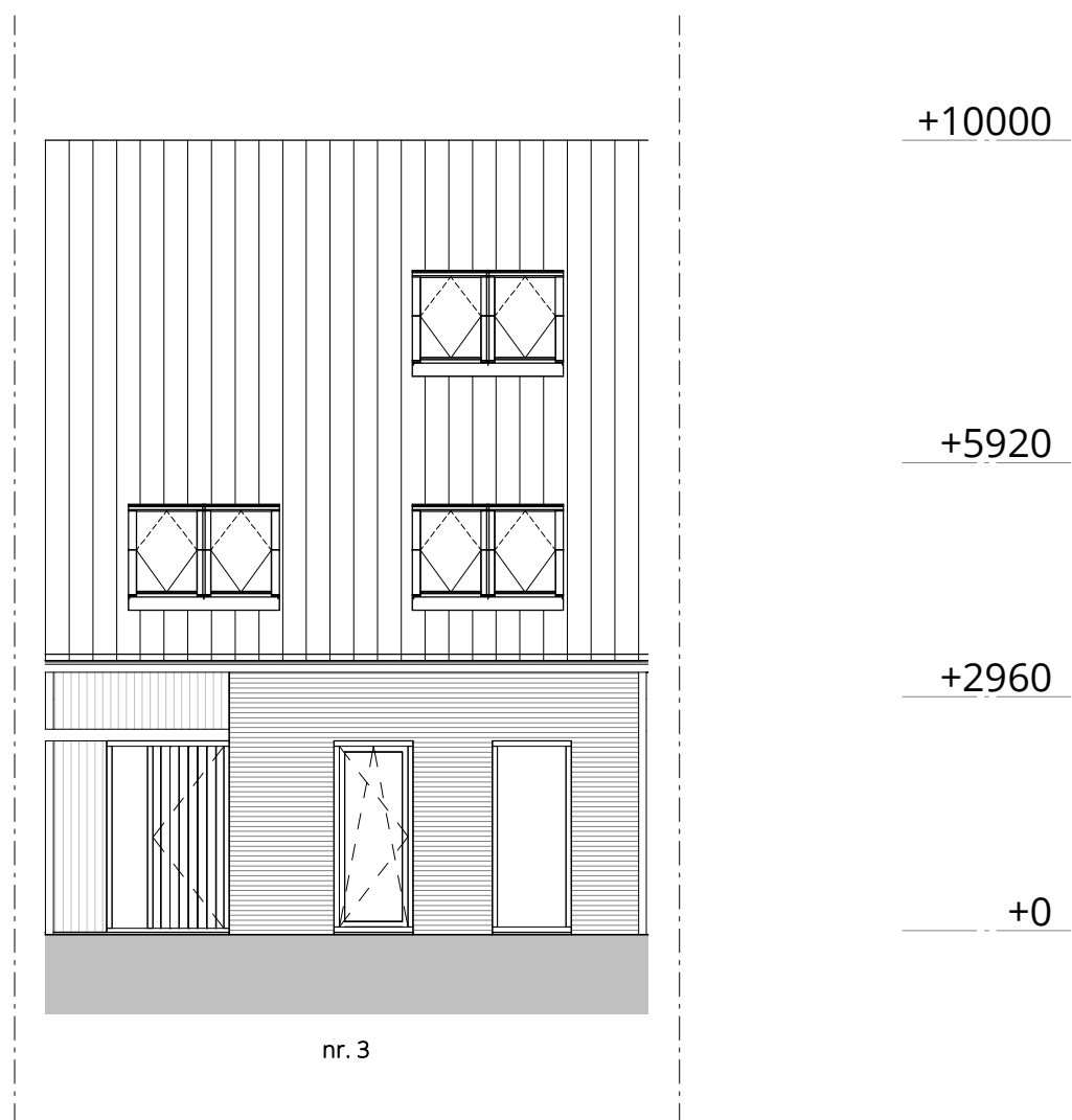
noordoost gevel
