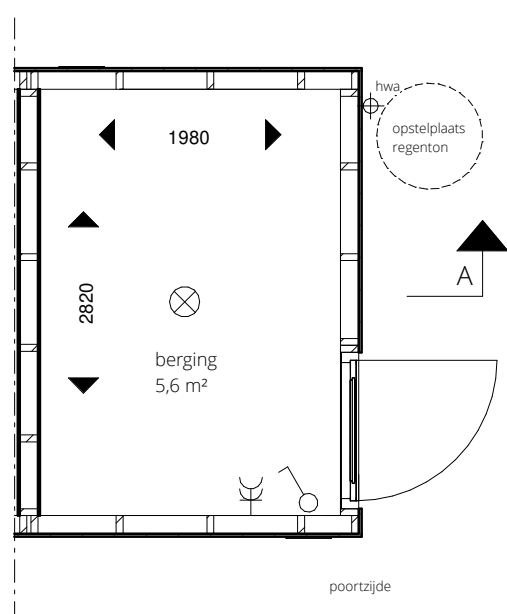
begane grond
