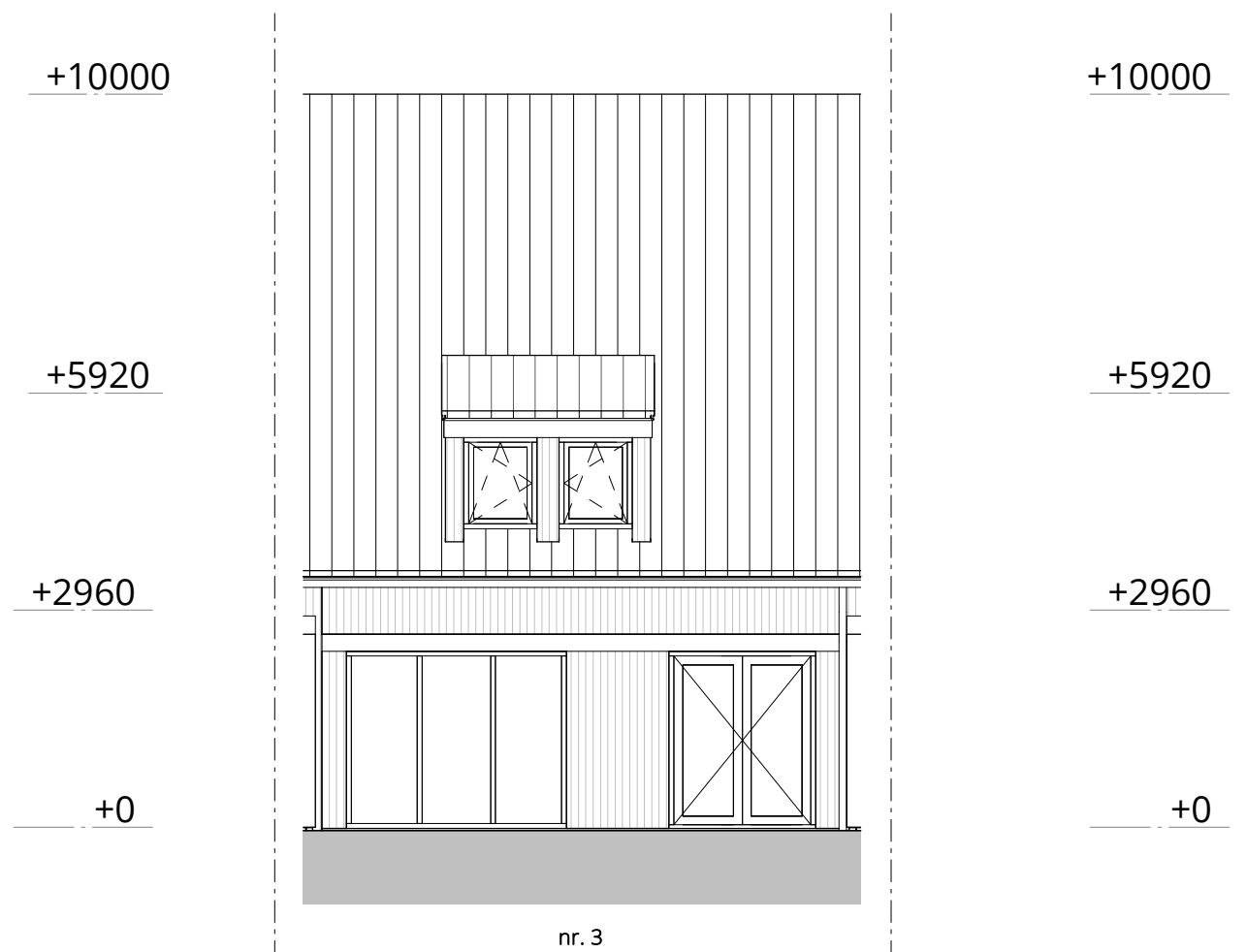
zuidwest gevel - optie dakkapel
