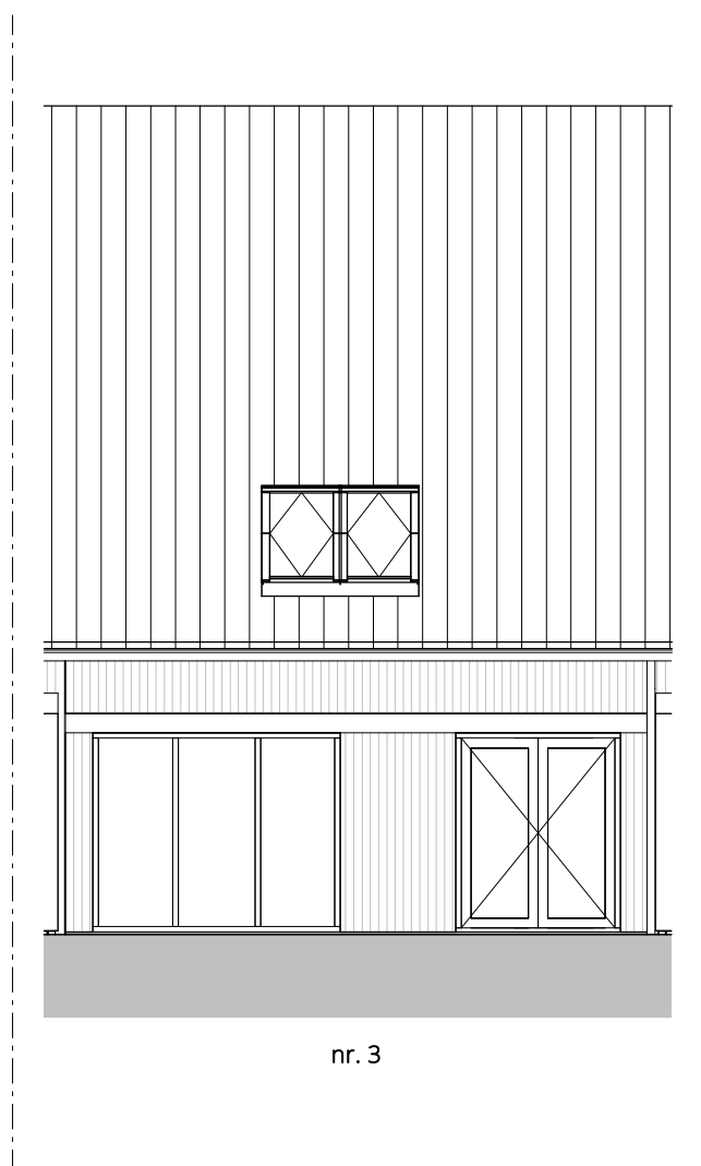
zuidwest gevel
