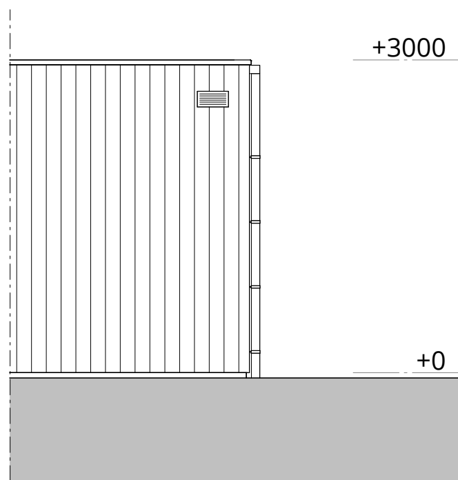
voorgevel
