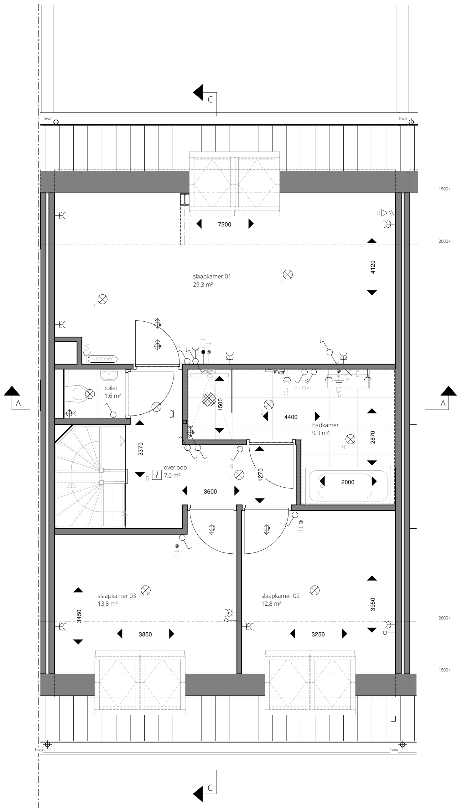
eerste verdieping
