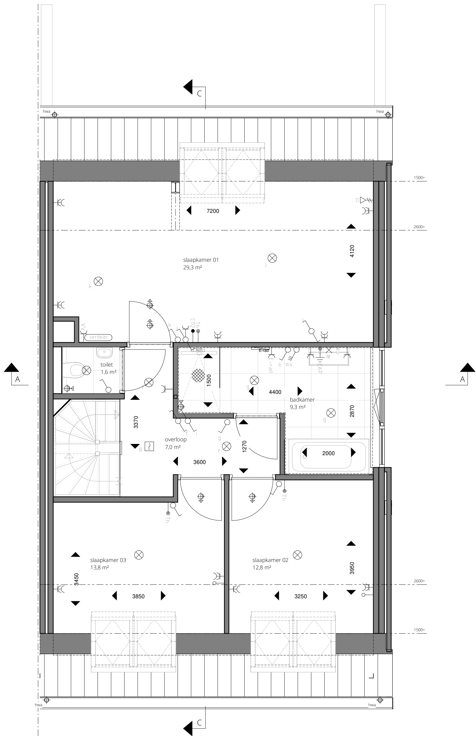
eerste verdieping
