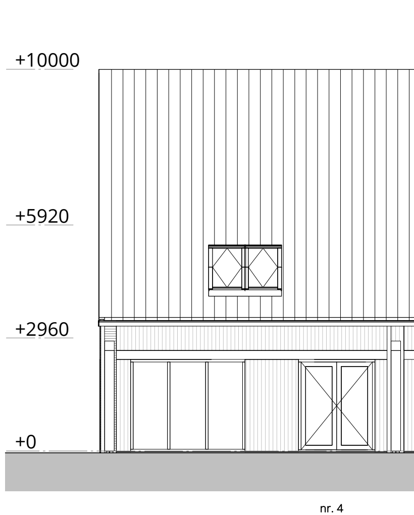
zuidwest gevel
