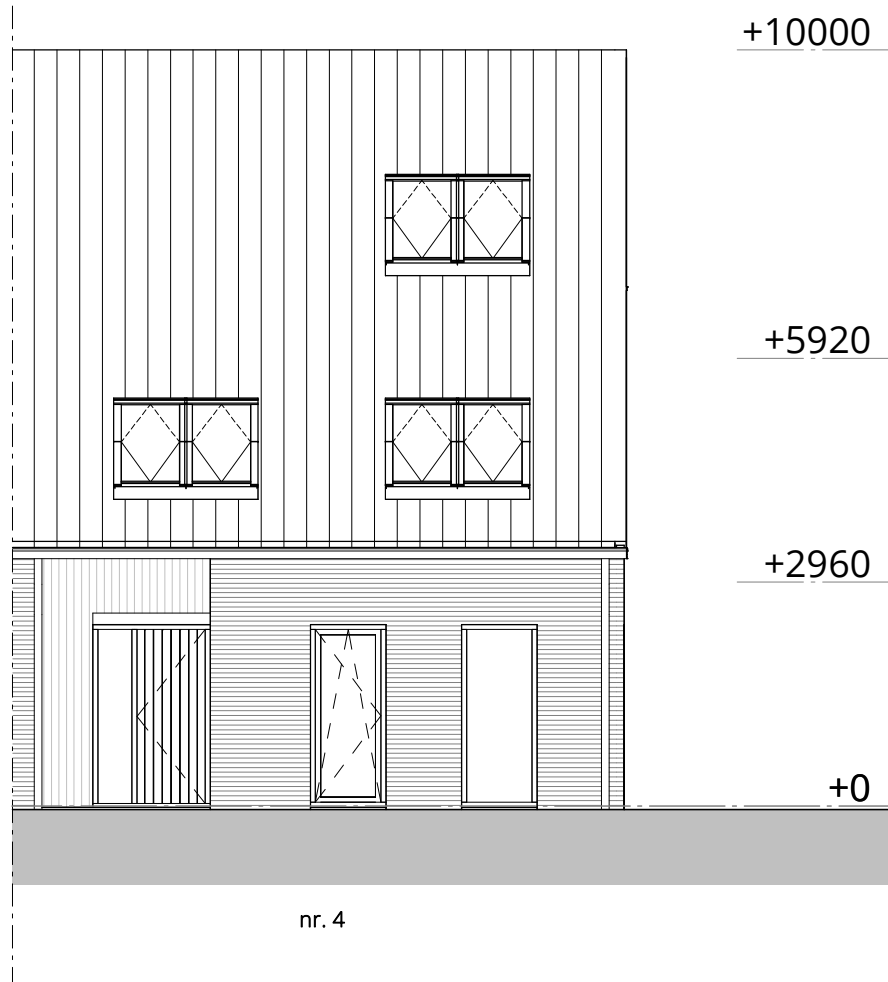
noordoost gevel
