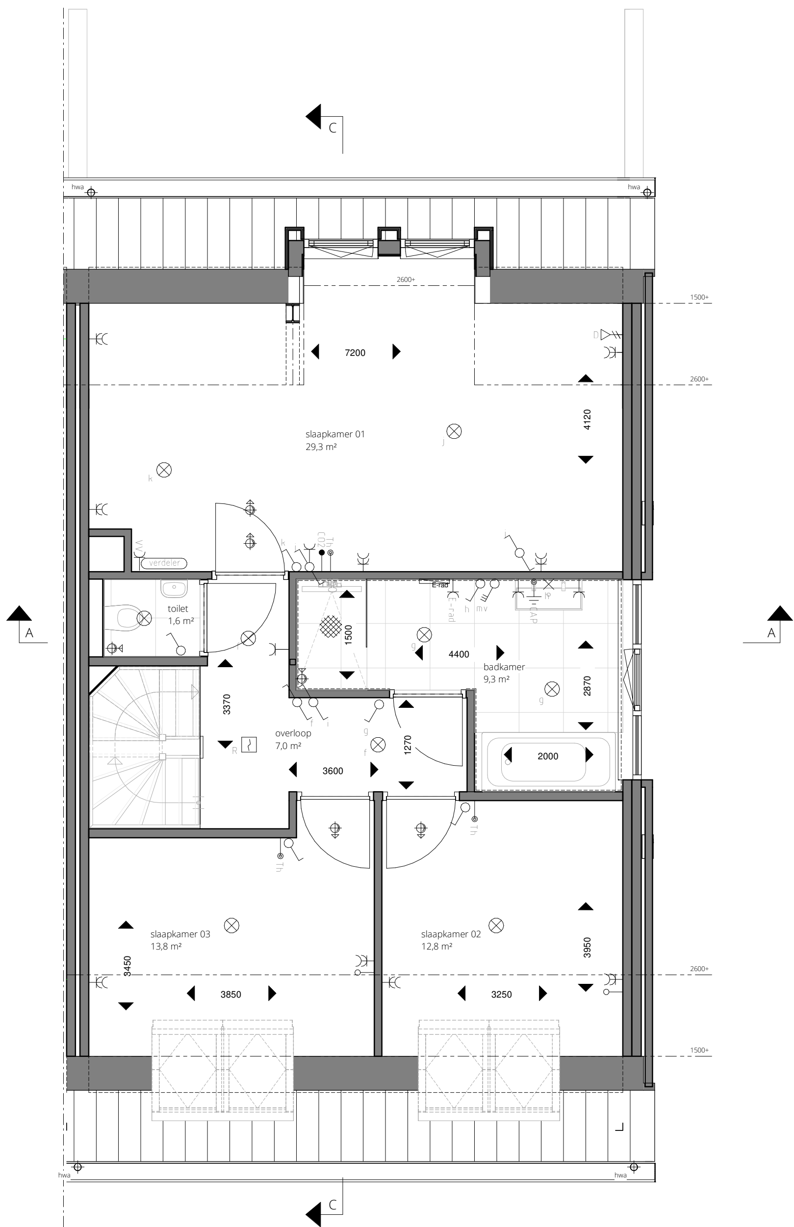
eerste verdieping optie dakkapel
