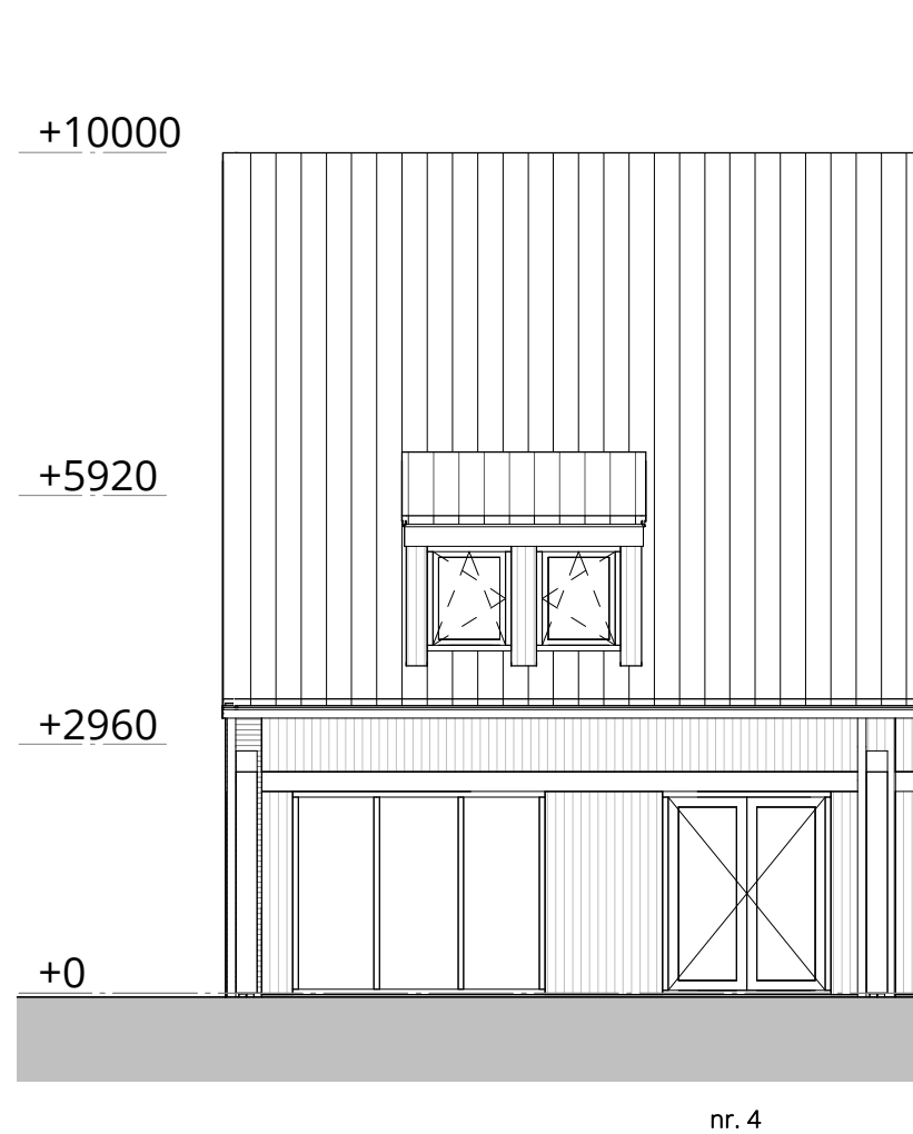
zuidwest gevel - optie dakkapel
