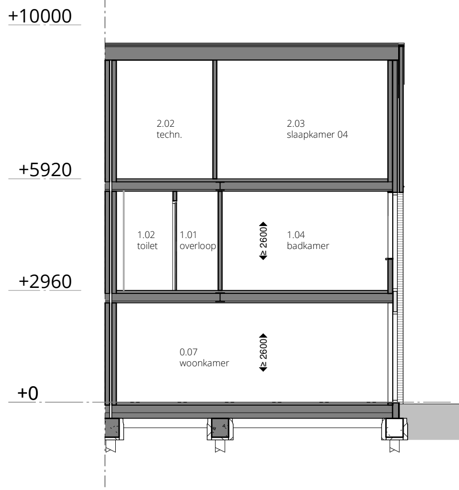
doorsnede A-A
