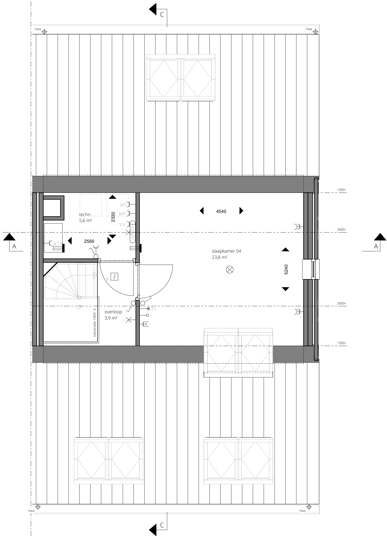
tweede verdieping
