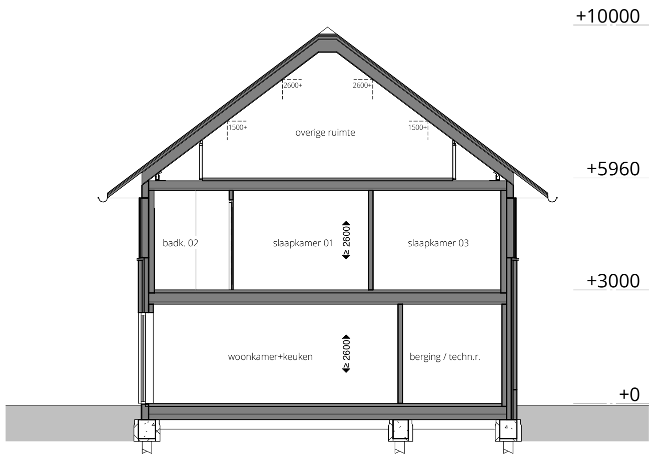
doorsnede A-A
