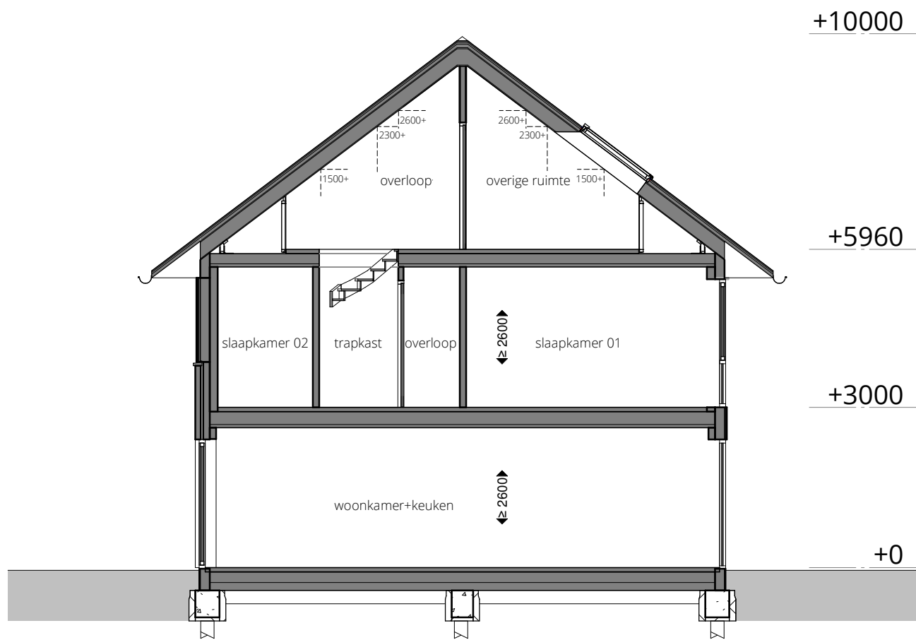
doorsnede B-B
