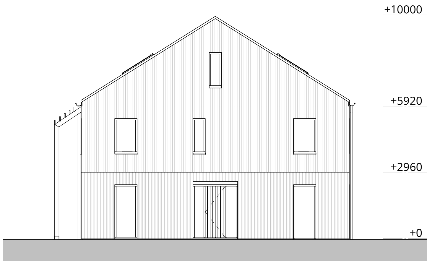
gevel noordoost
