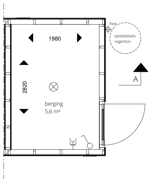
begane grond
