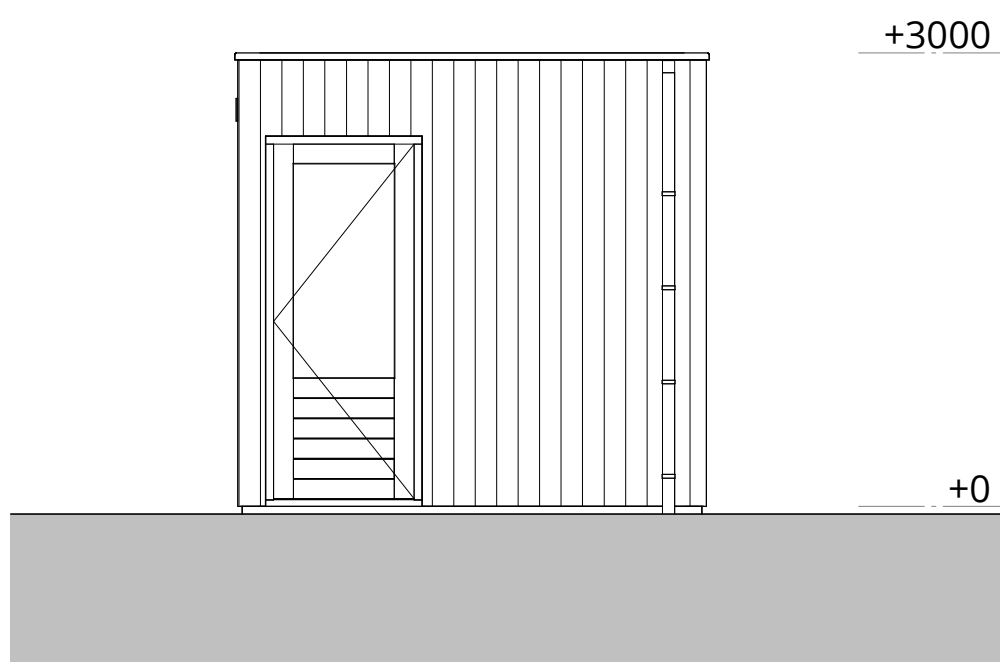
rechtergevel
