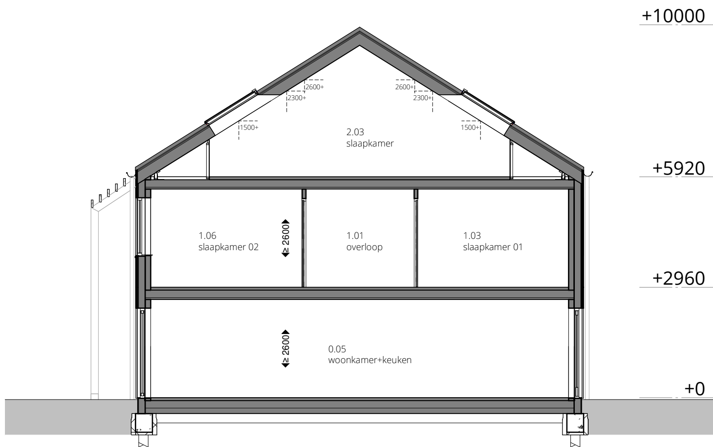
doorsnede B-B
