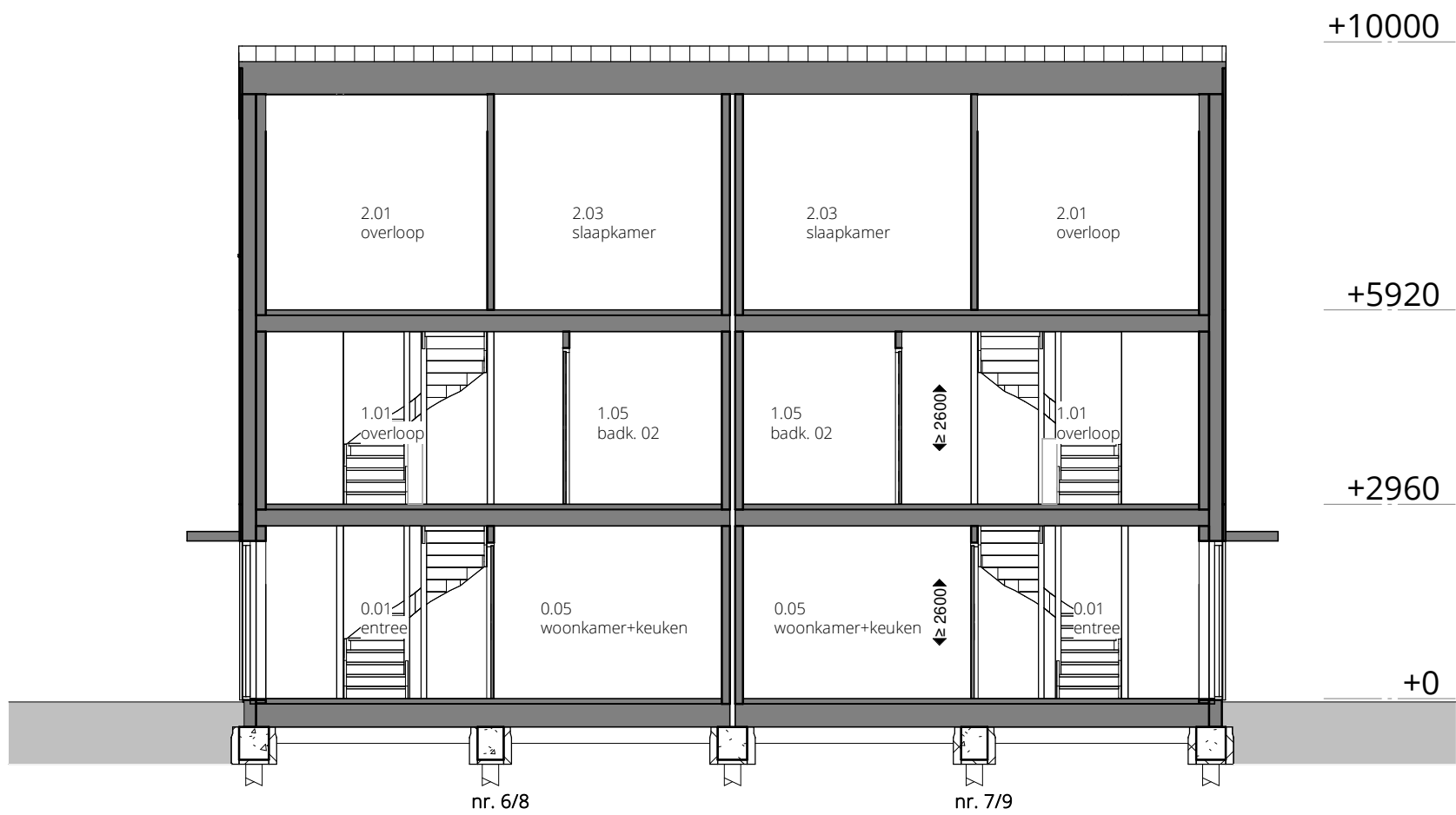
doorsnede A-A
