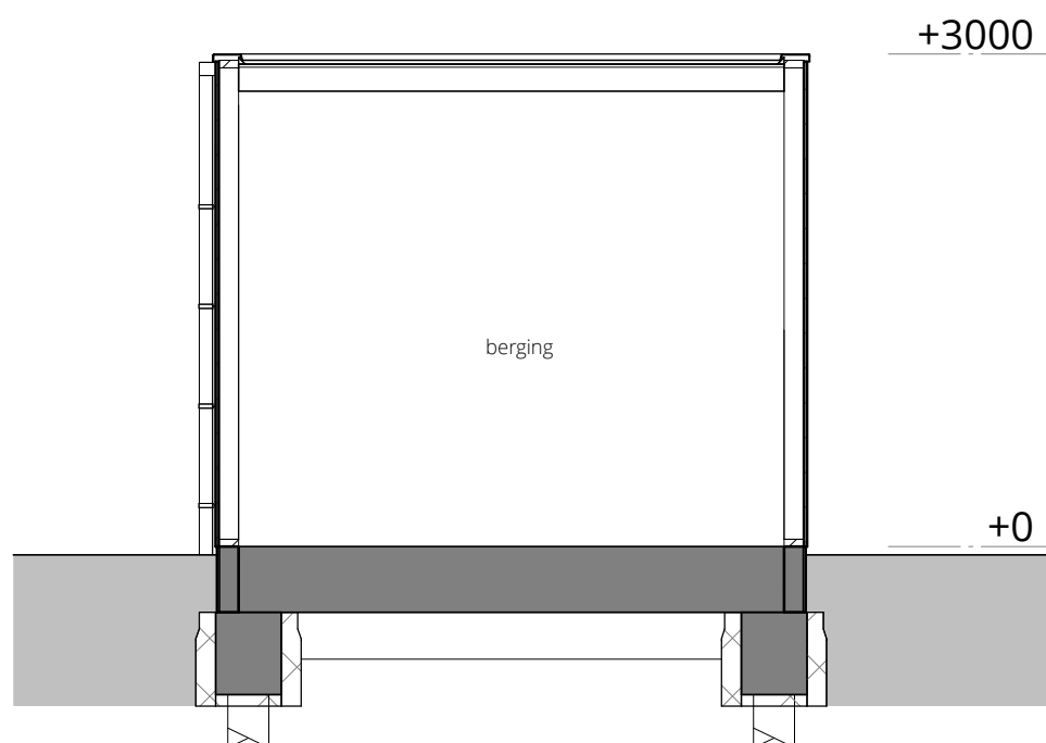
doorsnede A-A
