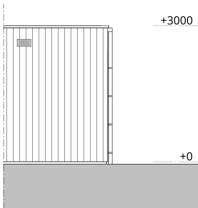
achtergevel
